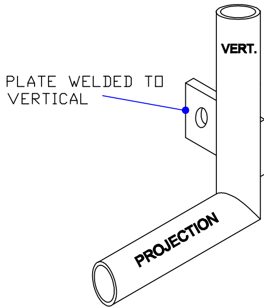
(VD-1r) VERTICAL DETAIL 1r
