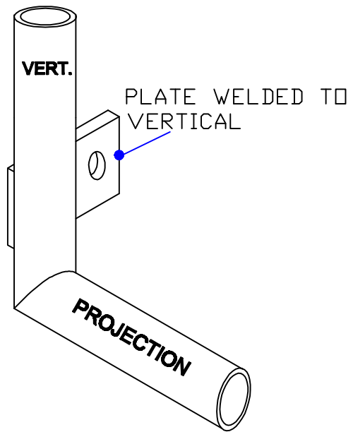
(VD-1r) VERTICAL DETAIL 1r
